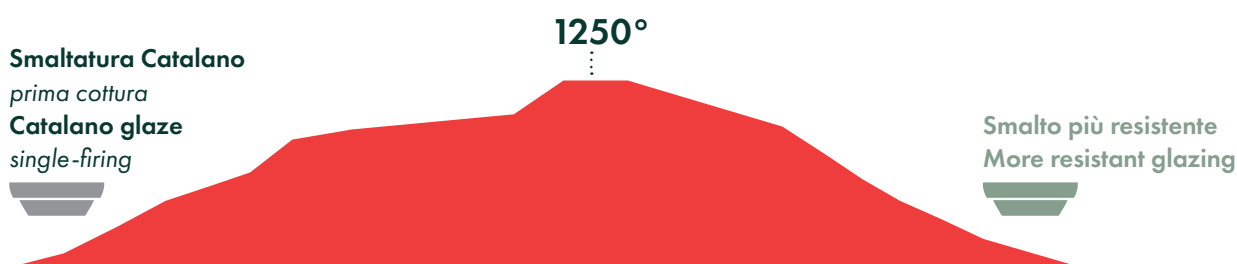
Curva di cottura Firing curve
